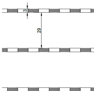
Schlitzbild 32/3 vorne
