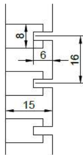
Querschnitt
